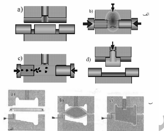
شکل ۱ الف) توالی عملیات در فرایند هیدروفرمینگ لوله ب) فرایند دبل بالچ تیوب هیدروفرمینگ [۳]
