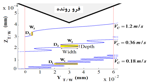
الف) نرخ پیشروی ثابت feed = 0.4 \text{ mm/rev} ، (D_1 < D_2 < D_3, W_1 > W_2 > W_3)
