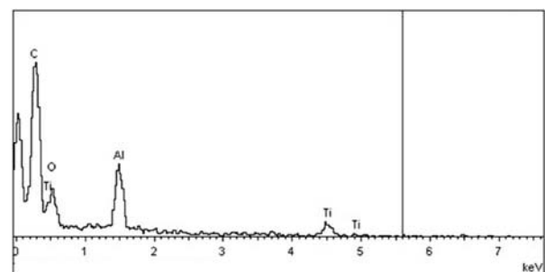
شکل ۹ آنالیز موضعی EDS مربوط به قسمت تیره رنگ در نمونه ماشینکاری شده با الکتروود مس
