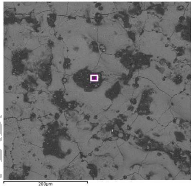
شکل ۸ آنالیز موضعی EDS بر روی قسمت تیره رنگ مشخص شده در تصویر BS-SEM
