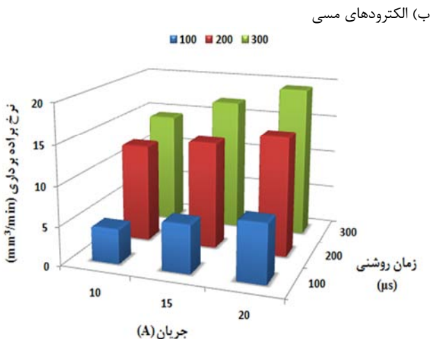
شکل ۱ نرخ براده‌برداری در ماشینکاری نمونه های TiAl با استفاده از سه نوع الکتروود ابزار
