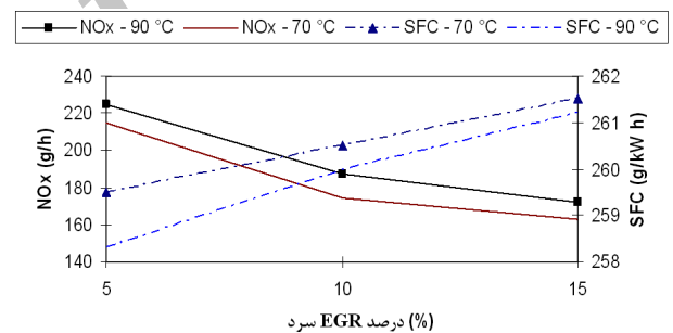
شکل ۴ تغییرات آلاینده NOx و مصرف سوخت ویژه در زاویه پاشش 8° BTDC به ازای تغییر در دمای خنک‌کاری و تغییر درصد EGR
