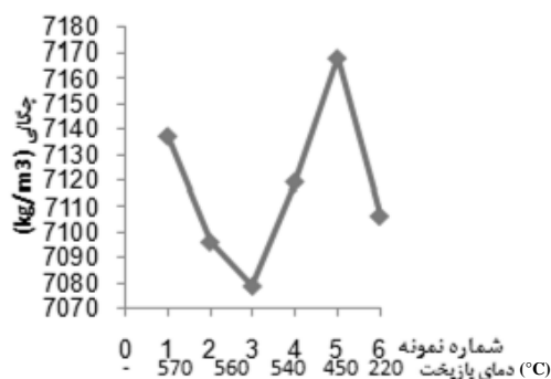
شکل ۸ تاثیر دمای بازیخت بر روی چگالی نمونه‌ها
