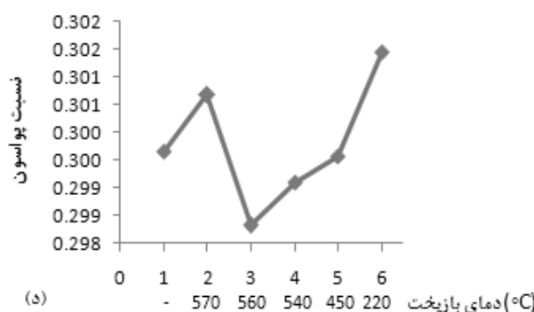
شکل ۷ تاثیر دمای بازیخت بر روی خواص مکانیکی نمونه‌های فولاد AISI D6: (الف) مدول برشی (ب) مدول یانگ (ج) مدول حجمی (د) نسبت پواسون
