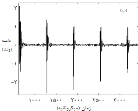
شکل ۳ نمونه‌ای از سیگنال‌های دریافتی از قطعه کار، (الف) موج طولی (ب) موج عرضی
