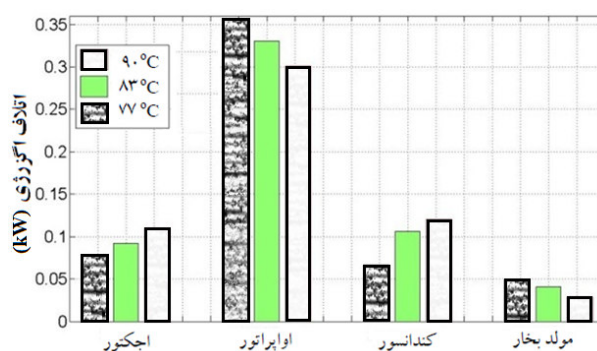
شکل ۱۳ تأثیر دمای مولد بخار بر روی اتلاف انرژی اجکتور در دماهای مختلف چرخه تبرید در دمای اوپراتور ۱۳/۵ درجه سلسیوس
