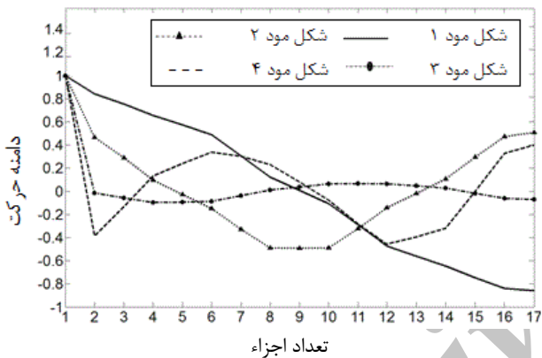
شکل ۱۴ مودهای اول تا چهارم مدل ۱۷ درجه آزادی میل‌لنگ پژو GLX
