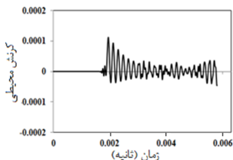
شکل ۵ نمودار کرنش محیطی بر حسب زمان در محل گنج ۵ (شبیه‌سازی عددی)
