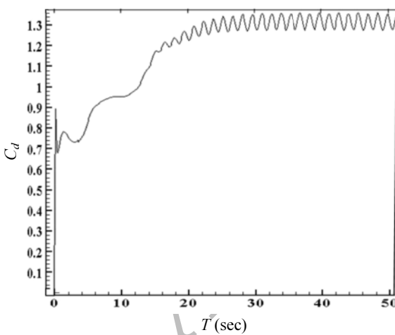
شکل ۵ نمودار تغییرات ضرایب درگ در پشت سیلندر اصلی در Re=200 در حالت عدم وجود سیلندر کنترلی
