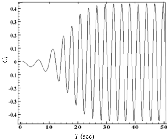
شکل ۴ نمودار تغییرات ضرایب لیفت در پشت سیلندر اصلی در Re=200 در حالت عدم وجود سیلندر کنترلی
