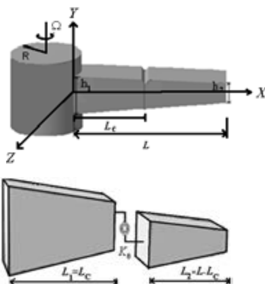
شکل ۱ تیر دورانی ترک‌دار با سطح مقطع متغیر
