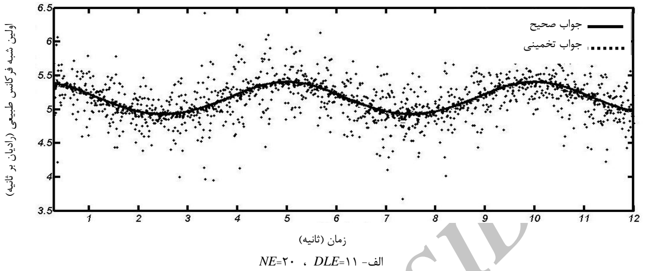
شکل ۵ مقدار انحراف جواب تخمین زده شده از جواب واقعی با تغییر تعداد آزمایش‌ها
