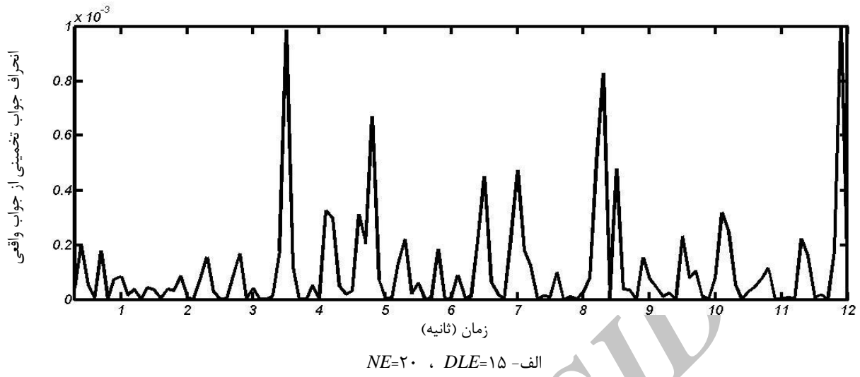
شکل ۲ فرکانس طبیعی اول سیستم به ازای داده‌هایی با طول متفاوت
