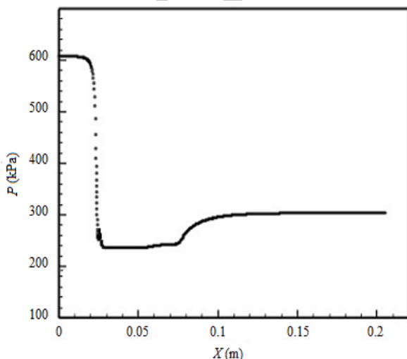
شکل ۸ تغییرات فشار استاتیکی جریان اولیه در طول خط تقارن اجکتور
