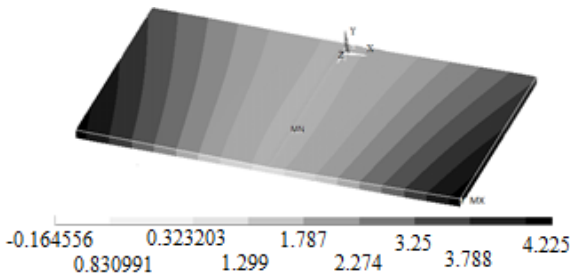
شکل ۵ توزیع تغییر شکل زاویه ای مدل المان محدود (اعداد بر حسب میلی متر)
