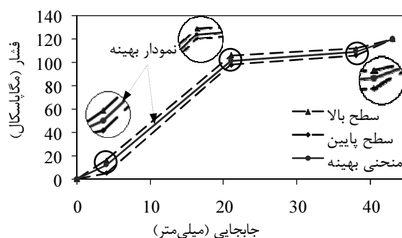
شکل ۱۱ مقدار بهینه حاصل از حل مدل نسبت به مقادیر مرزی
