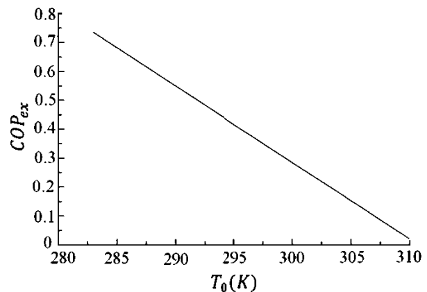
شکل ۱۱ نمودار ضریب عملکرد آگزرتیک چرخه میسوتسنکو
