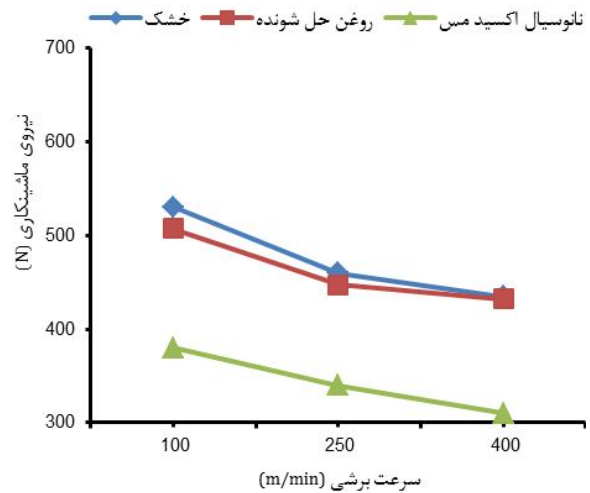
شکل ۹ تأثیر نانوسیال اکسید مس بر روی نیروی ماشین کاری در سرعت‌های برشی و شرایط محیطی مختلف ( \alpha_p=0.6 \text{ mm} و f=0.1 \text{ mm/rev} )
