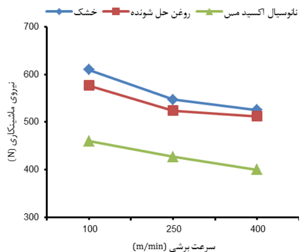
شکل ۱۰ تأثیر نانوسیال اکسید مس بر روی نیروی ماشین کاری در سرعت‌های برشی و شرایط محیطی مختلف ( \alpha_p=0.6 \text{ mm} و f=0.15 \text{ mm/rev} )
