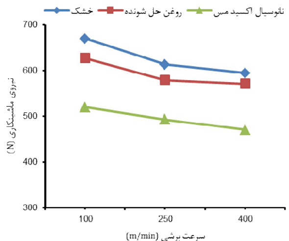
شکل ۱۱ تأثیر نانوسیال اکسید مس بر روی نیروی ماشین کاری در سرعت‌های برشی و شرایط محیطی مختلف ( \alpha_p=0.6 \text{ mm} و f=0.2 \text{ mm/rev} )
