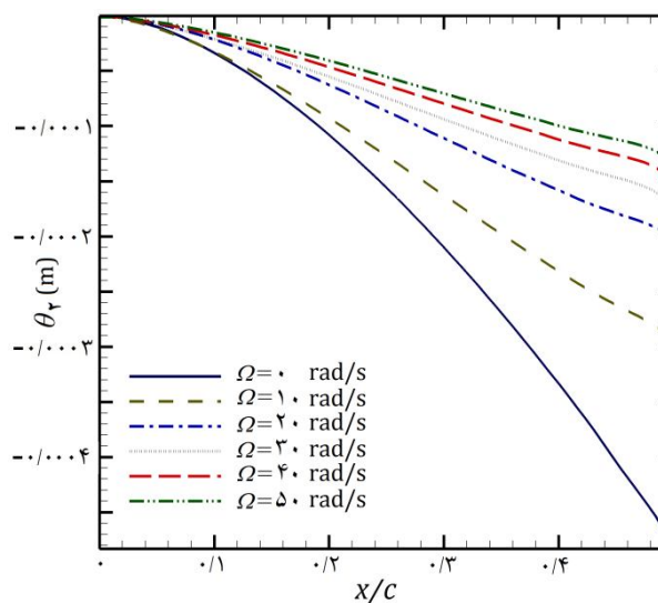
شکل ۲۰ تغییرات ضخامت مومنوم شعاعی در سرعت‌های چرخش متفاوت
