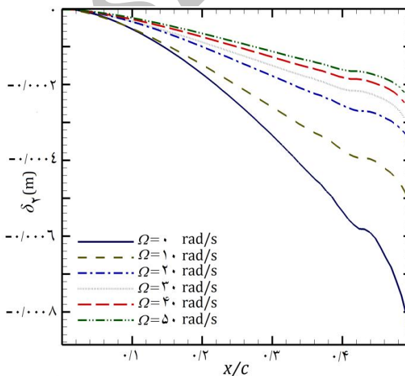
شکل ۱۹ تغییرات ضخامت جابجایی شعاعی در سرعت‌های چرخش متفاوت
