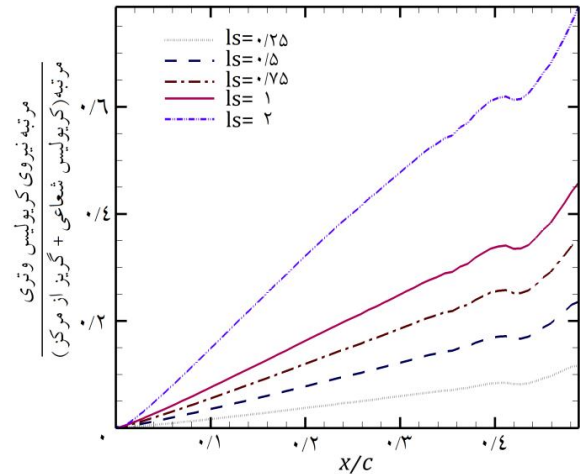
شکل ۲۱ نسبت مرتبه جمله کرپولیس وتری به مرتبه جملات کرپولیس شعاعی و گریز از مرکز
