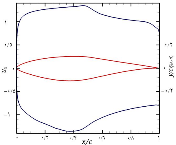
شکل ۱۶ توزیع سرعت غیر لزوج بر روی پره
