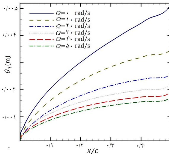
شکل ۱۸ تغییرات ضخامت مومنوم و تری در سرعت‌های چرخش متفاوت
