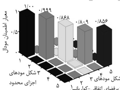
ت) معیار اطمینان مودال با اضافه شدن ۲۰٪ نویز-شاخص پیشنهادی
