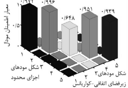
شکل ۱۵ (ب) معیار اطمینان مودال با اضافه شدن ۱۲٪ نویز-شاخص همبستگی
