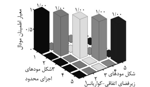
شکل ۸ مقایسه شکل مودهای محاسبه شده به روش زیر فضاهای اتفاقی بر مبنای کواریانس و روش اجزای محدود-شاخص همبستگی
