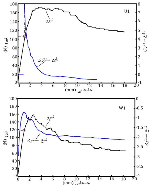
شکل 18 رفتار تابع سنتری برای نمونه‌های U1 و W1 و تعیین مقدار بار بحرانی با این روش
