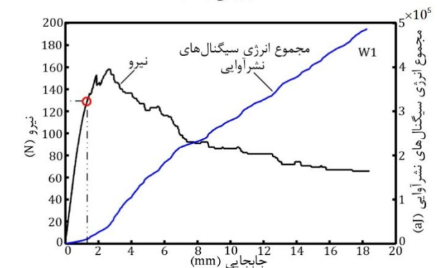
شکل 15 تعیین مقدار بار بحرانی با روش افزایش ناگهانی مجموع انرژی نشر آوایی برای نمونه‌های U1 و W1
