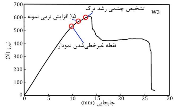
شکل 14 مقادیر بار بحرانی بدست آمده با روش‌های مختلف برای نمونه‌های U3 و W3
