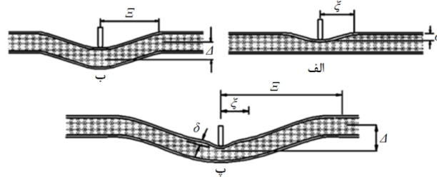
شکل ۶ فرورفتگی موضعی، (ب) تغییر شکل خمشی-برشی سراسری و (پ) تغییر شکل‌های موضعی و سراسری [۶]
