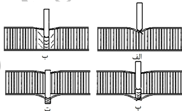
شکل ۷ شکست رویه جلویی، (ب) شکست برشی و له شدن موضعی هسته، (پ) گسیختگی رویه پشتی و (ت) خروج پرتابه و تشکیل پلاگ
