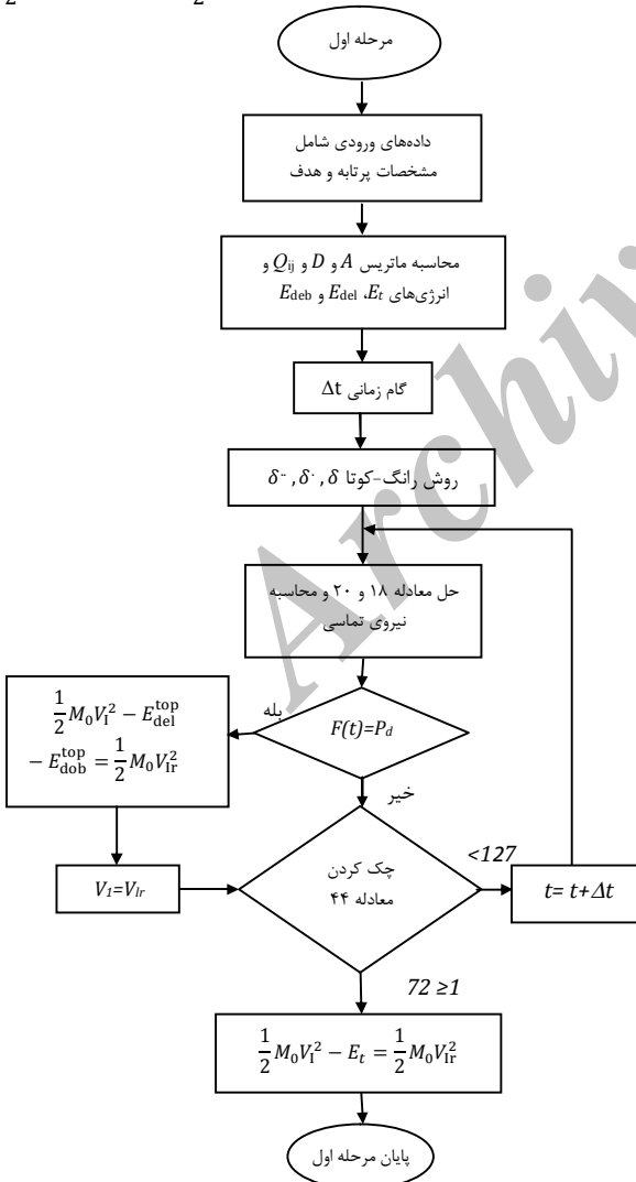
شکل ۱۰ فلورچارت مرحله اول حل
