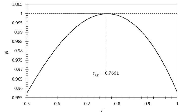
شکل 5 تغییرات \phi بر حسب \bar{r} را برای n = n_{cr} و \Omega = 1.39308 < \Omega_{cr}
