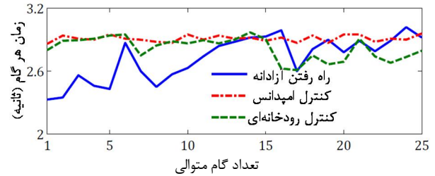
شکل 15 دوره‌ی زمانی گام بیمار در راه رفتن آزادانه، به کمک کنترل امیدانس و به کمک کنترل رودخانه‌ای
