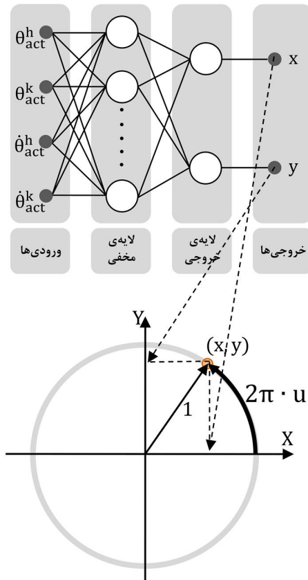
شکل 3 در الگوریتم تشخیص فاز حرکت، شبکه عصبی زاویه و سرعت زاویه‌ای واقعی مفاصل را دریافت می‌کند و فاز حرکت (مقدار u ) را تخمین می‌زند
