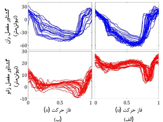
شکل 16 گشتاورهای اعمالی به مفاصل ران و زانو بیمار در دو حالت (الف) کنترل امیدانس و (ب) کنترل رودخانه‌ای
