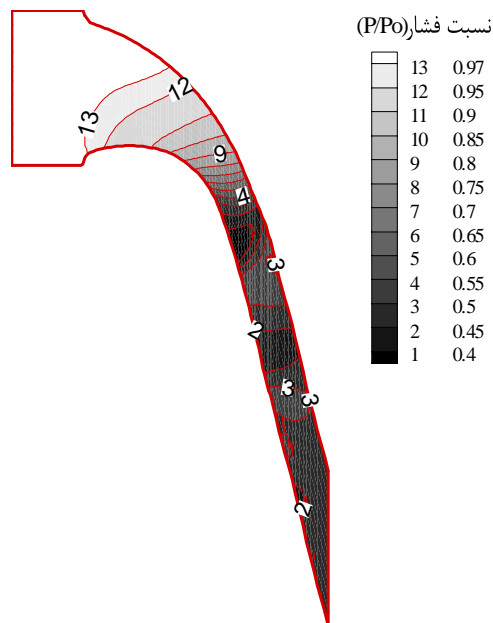
شکل 3 خطوط هم‌فشار برای نسبت فشار استاتیک به فشار سکون اولیه در طول پره
