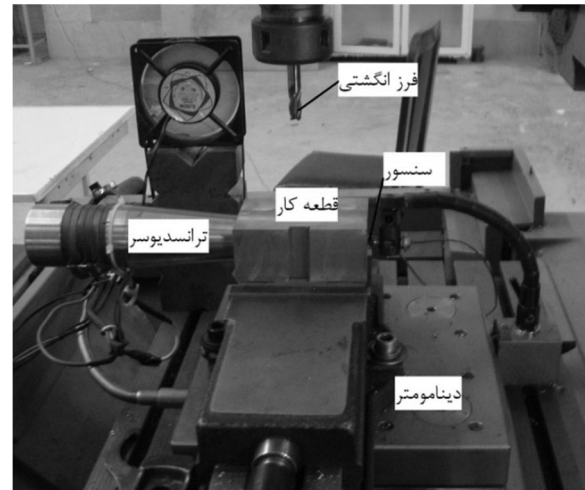
شکل 6 تنظیم تجربی برای آزمایش های فرزکاری معمولی و آلتراسونیک
