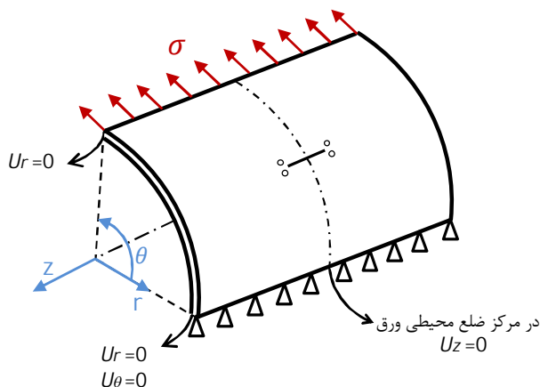
شکل 3 بارگذاری و شرایط مرزی مدل اجزا محدود
