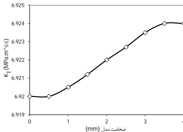
شکل 6 تغییرات ضریب شدت تنش مد یک در راستای ضخامت ورق با شعاع انحنای r = 1m
