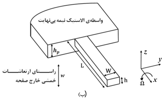
شکل 6 الف- واسطه الاستیک نیمه‌بی‌نهایت (تکیه‌گاه) به همراه پارامترهای مورد استفاده در مطالعه اتلاف تکیه‌گاه ب- واسطه الاستیک نیمه‌بی‌نهایت و نیرو و گشتاورهای اعمالی در نقطه اتصال تیر به تکیه‌گاه [10]
