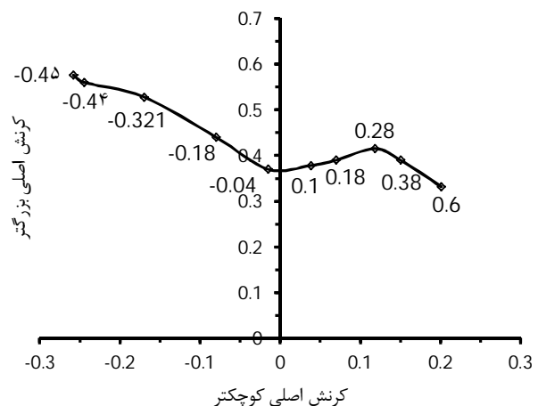
شکل 16 منحنی حد شکل‌دهی لوله فولادی زنگ‌نزن 304، حاصل از آزمایش‌های تجربی (اعداد روی نمودار بیان‌کننده نسبت کرنش \beta است)
