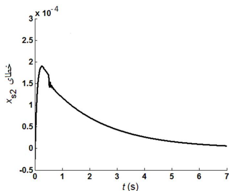
شکل 11 خطای تعقیب مسیر حرکت جسم
