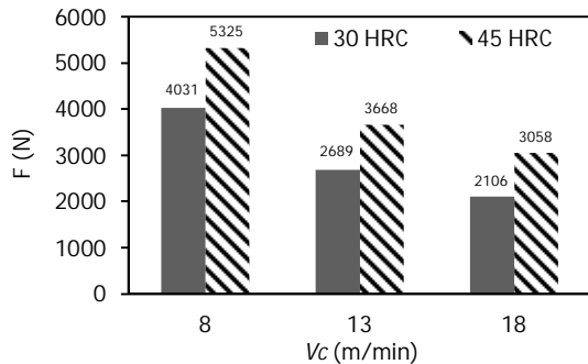
شکل 8 تأثیر تغییرات سرعت برشی بر نیروی ماشین کاری
