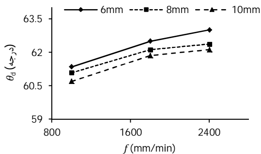
شکل 16 منحنی زاویه حد شکل‌پذیری لایه بیرونی بر حسب سرعت پیشروی در حالت AS و z=0/25 mm
