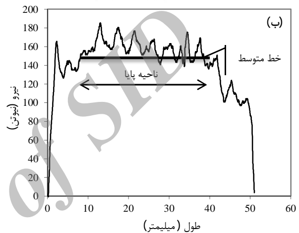
شکل 2 تست پوست‌کنی: الف- شماتیک تست؛ ب- نمودار نیروی پوست‌کنی در برابر طول پوست‌کنی شده
