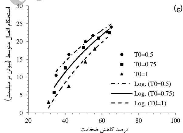
شکل 6 اثر درصد کاهش ضخامت بر استحکام اتصال در مقادیر مختلف ضخامت اولیه آلومینیوم T_0 ؛ میزان کار سرد اولیه آلومینیوم برابر الف - صفر، ب-17% و ج-37/5%.
