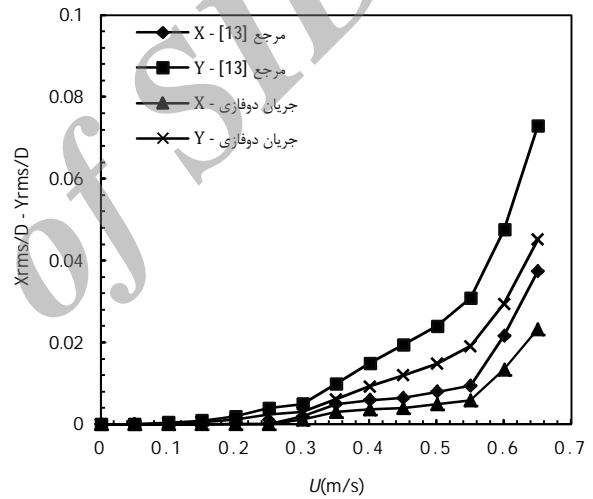
شکل 16 دامنه نوسان در جهت X و Y برای حالت تک سیلندر متحرک (دسته سیلندر 1) - کسر حجمی 0/1
