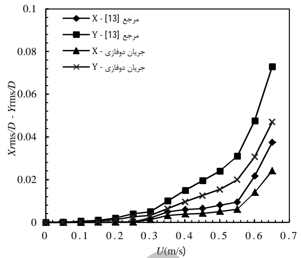
شکل 15 دامنه نوسان در جهت X و Y برای حالت تک سیلندر متحرک (دسته سیلندر 1) - کسر حجمی 0/08
