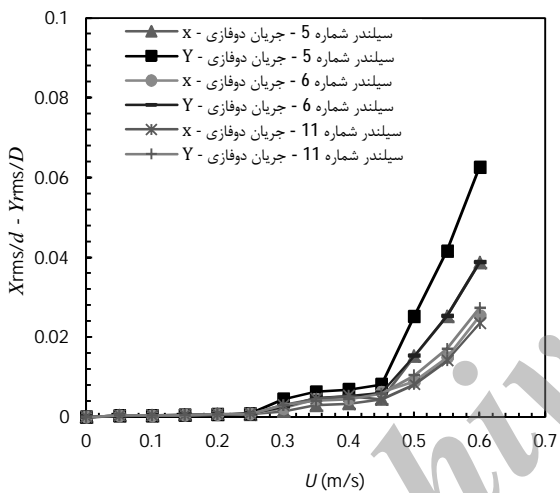
شکل 19 دامنه نوسان در جهت X و Y برای حالت سه سیلندر متحرک (دسته سیلندر 3) - کسر حجمی 0/04
