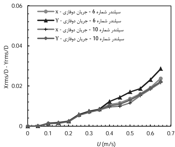
شکل 21 دامنه نوسان در جهت x و y برای حالت چهار سیلندر متحرک (دسته سیلندر 4) - کسر حجمی 0/06 - سیلندر شماره 6 و 10
