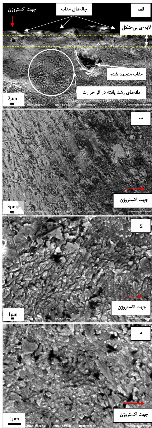
شکل 14 تصویر FE-SEM از ریز ساختار زیر لایه‌ی عمق - الف) 60µm (ب) 200µm (ج) 400µm (د) 900µm
