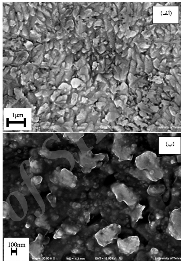
شکل 18 تصویر FE-SEM از ریز ساختار مس تولید شده توسط قالب 110^\circ = \theta در (الف) پاس 4 (ب) پاس 8
