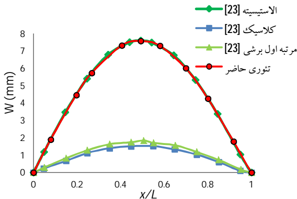
شکل 8 نمودار جایجایی رویه بالایی در طول تیر ساندویچی با استفاده از تئوری‌های مختلف
