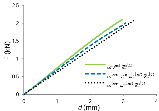
شکل 6 نمودار نیرو - جایجایی مقایسه‌ای برای تیرهای کوتاه ساندویچی
