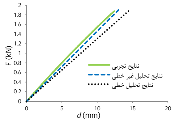
شکل 7 نمودار نیرو - جایجایی مقایسه‌ای برای تیرهای بلند ساندویچی
