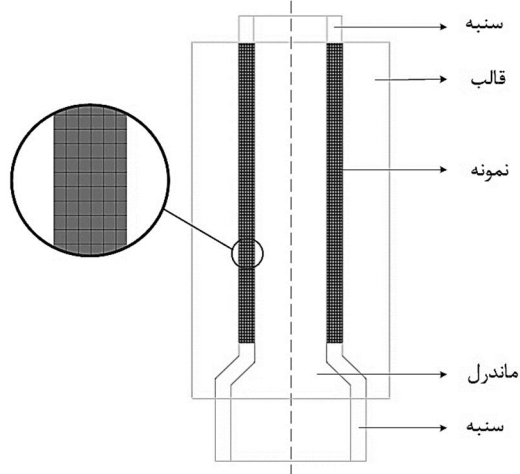
شکل 3 نمونه‌ای از مدل ساخته شده شامل لوله مش‌بندی شده
