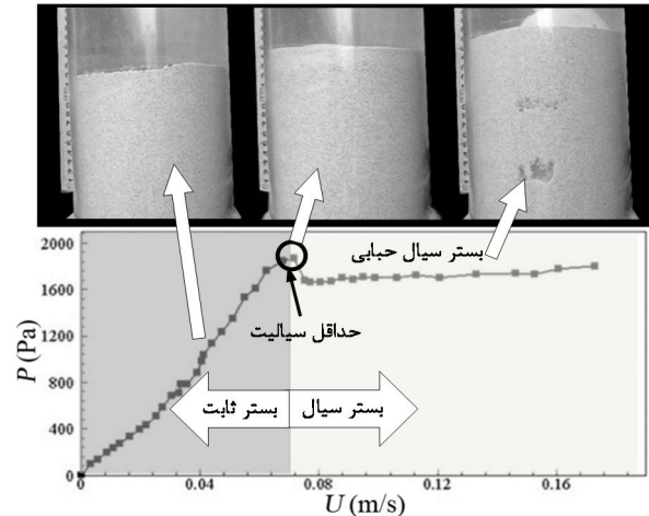
شکل 3 رفتار فشار بستر در برابر سرعت گازهای ورودی
