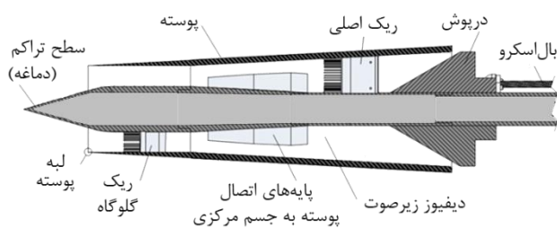
شکل ۳ نمای شماتیک مدل و متعلقات آن
