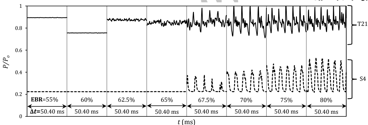
شکل ۸ فشار ثبت شده توسط حسگر S4 و T21 برحسب زمان و نسبت انسداد در M_{\infty}=2/0 (داده‌های ثبت شده در ۵۰/۴۰ میلی‌ثانیه‌ی ابتدایی برای هر نسبت انسداد)
