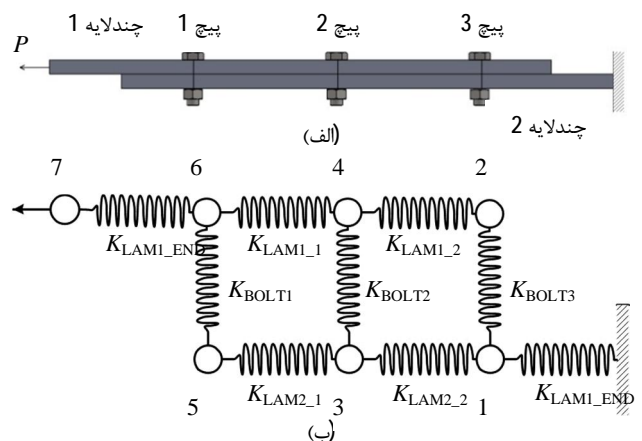
شکل 4 اتصال تک‌لایه سه پیچه: الف- ساختار اتصال. ب- مدل‌سازی جرم-فنر متناظر
