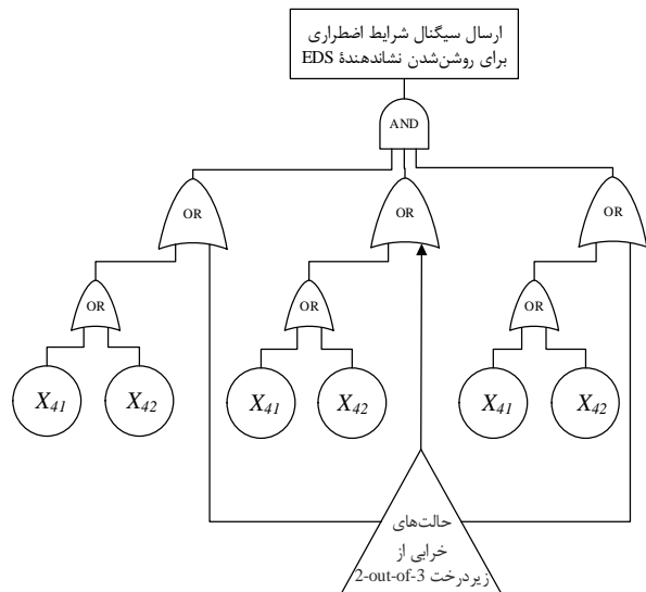
شکل 11 ساختار ترکیبی درخت خطای سیستم چندحالتی غیرمنسجم تشخیص شرایط اضطراری یک فضایما
