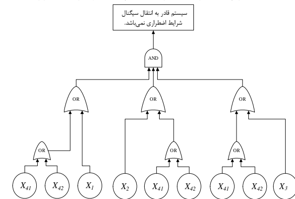
شکل 2 درخت خطای سیستم تشخیص شرایط اضطراری
