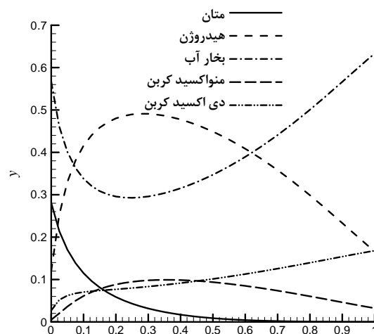
شکل 7 توزیع کسر مولی گونه‌ها در طول کانال سوخت
