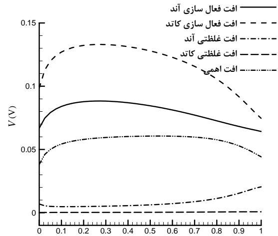
شکل 10 منحنی توزیع افت های مختلف در طول پیل
