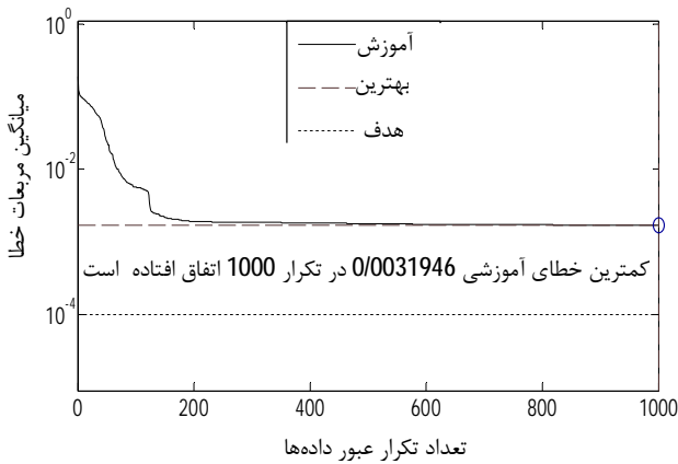
شکل 19 همگرایی خطا در آموزش شبکه
