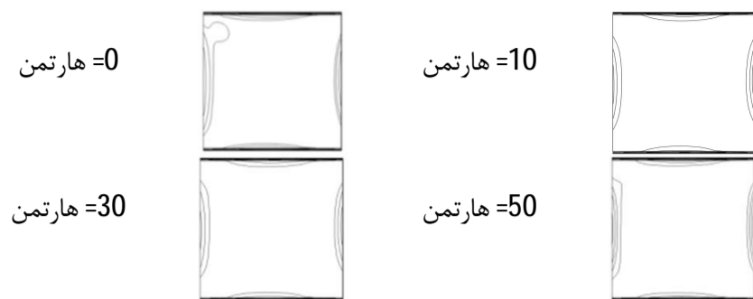
شکل 7 کانتورهای تولید آنتروپی کل در عدد رایلی 10^3 ، زاویه انحراف 0^\circ و اعداد هارتمن مختلف (نانوسیال آب - آلومینا، 5%).
