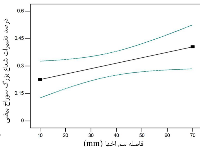
شکل 20 درصد تغییرات شعاع بزرگ سوراخ بیضی نسبت به فاصله سوراخها
