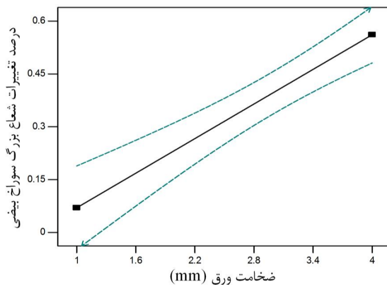
شکل 21 درصد تغییرات شعاع بزرگ سوراخ بیضی نسبت به ضخامت ورق
