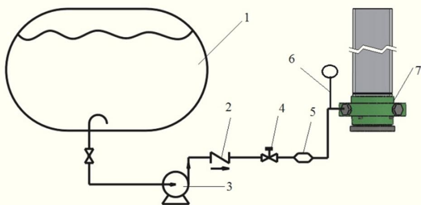
شکل 7 شمایی از مدار تست
