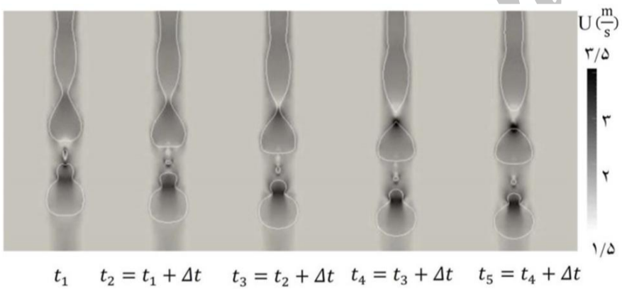
شکل 12 کانتور سرعت بر حسب \frac{m}{s} در لحظه شکست جت برای مقادیر حداکثر و حداکثر سرعت در هر لحظه ( \Delta t = 10^{-4} s )
