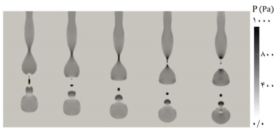
شکل 11 کانتور فشار بر حسب پاسکال در لحظه شکست جت برای مقادیر حداکثر و حداقل فشار در هر لحظه ( \Delta t = 10^{-4} s )
