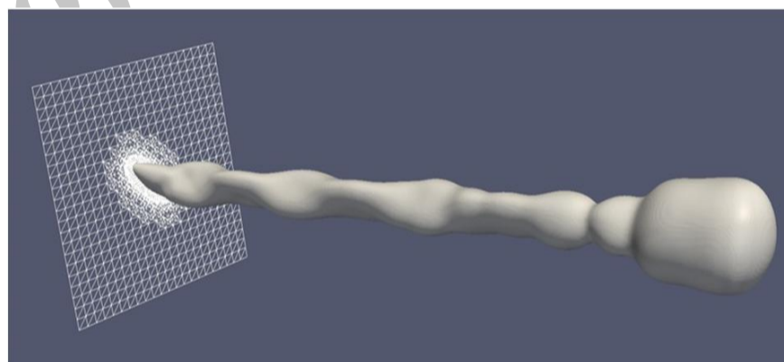
شکل 5 تصویر سه بعدی پدیده تغییر محور حاصل از شبیه سازی
