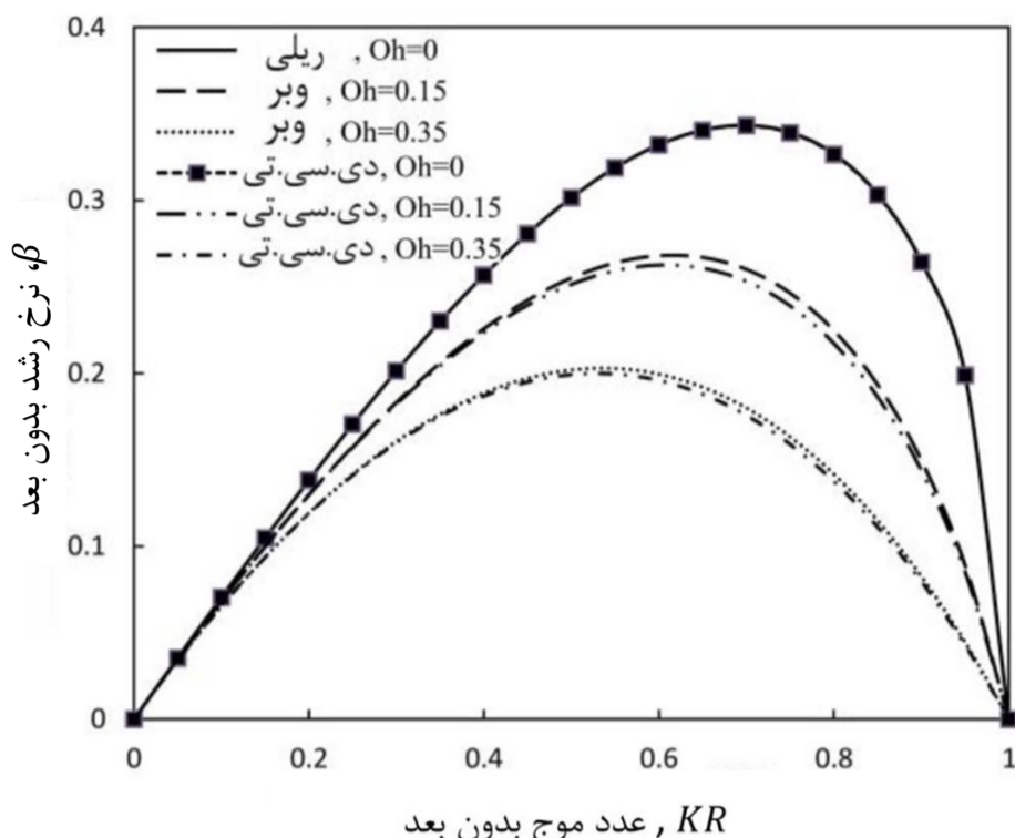
شکل 3 نرخ رشد بدون بعد بر حسب عدد موج بدون بعد برای جریان لزوج و غیر لزوج [21]
