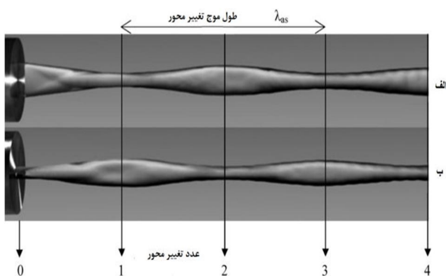
شکل 1 تصویر شماتیک از تخلیه جت بیضوی از حفره ای بیضوی (الف) شکل جت با حضور روی محور اصلی (ب) شکل جت با حضور روی محور فرعی [28]
