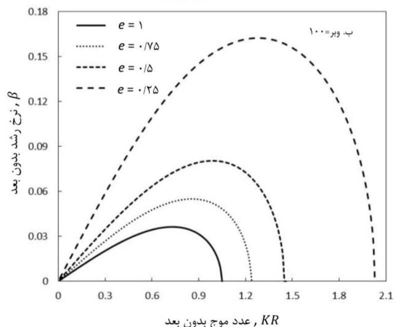
شکل 2 نرخ رشد بدون بعد بر حسب عدد موج بدون بعد برای الف) عدد ویر 10 ب) عدد ویر 100 [21]
