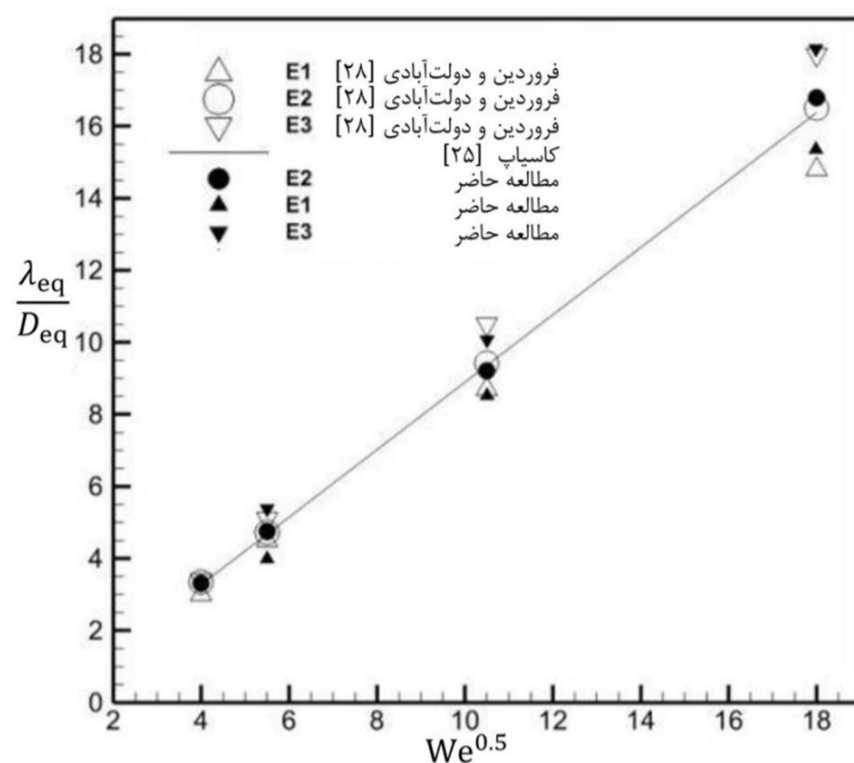
شکل 13 تغییرات طول موج تغییر محور بر حسب عدد وبر برای اریفیس E1, E2, E3
