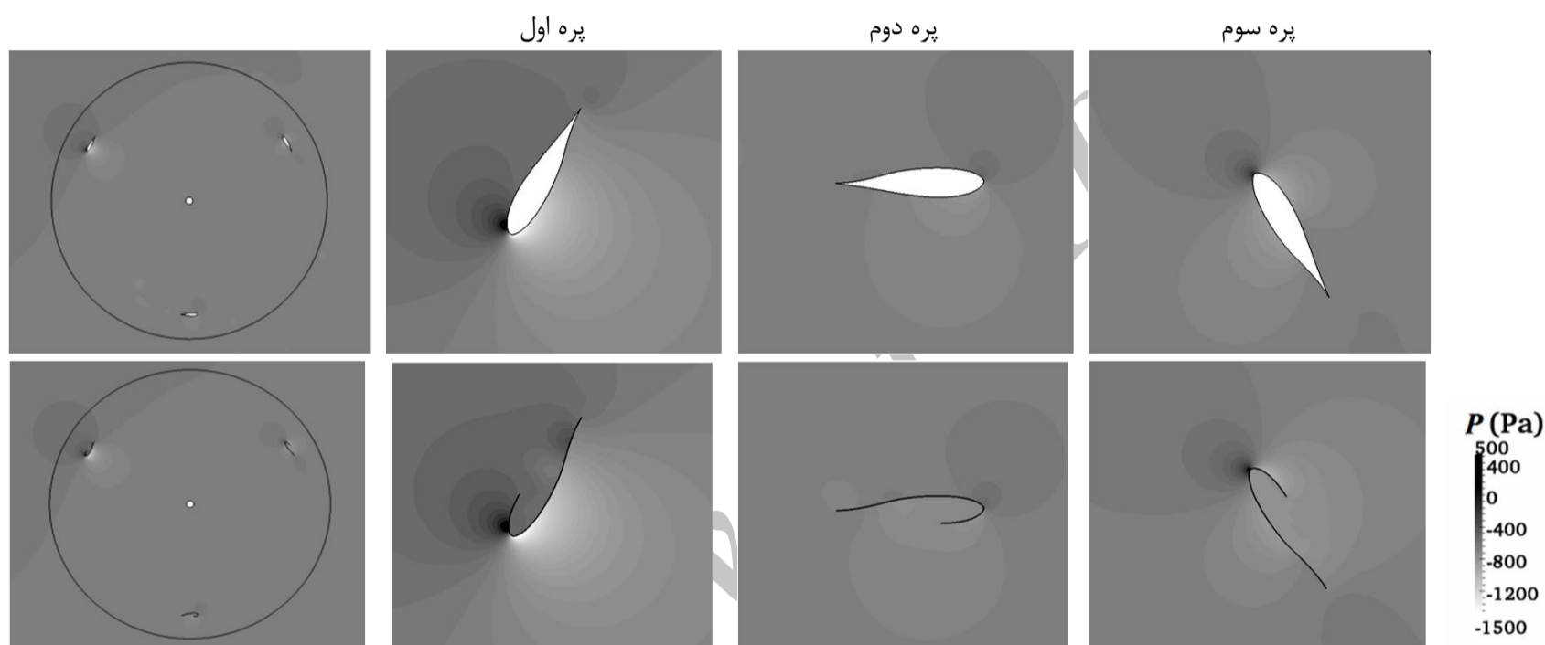
شکل 22 میدان فشار حول روتور و پره‌ها پس از رسیدن به حالت پایا در یک دور کامل برای پره با ایرفویل Du 06-W-200 و Du 33-J در سرعت نوک بهینه
