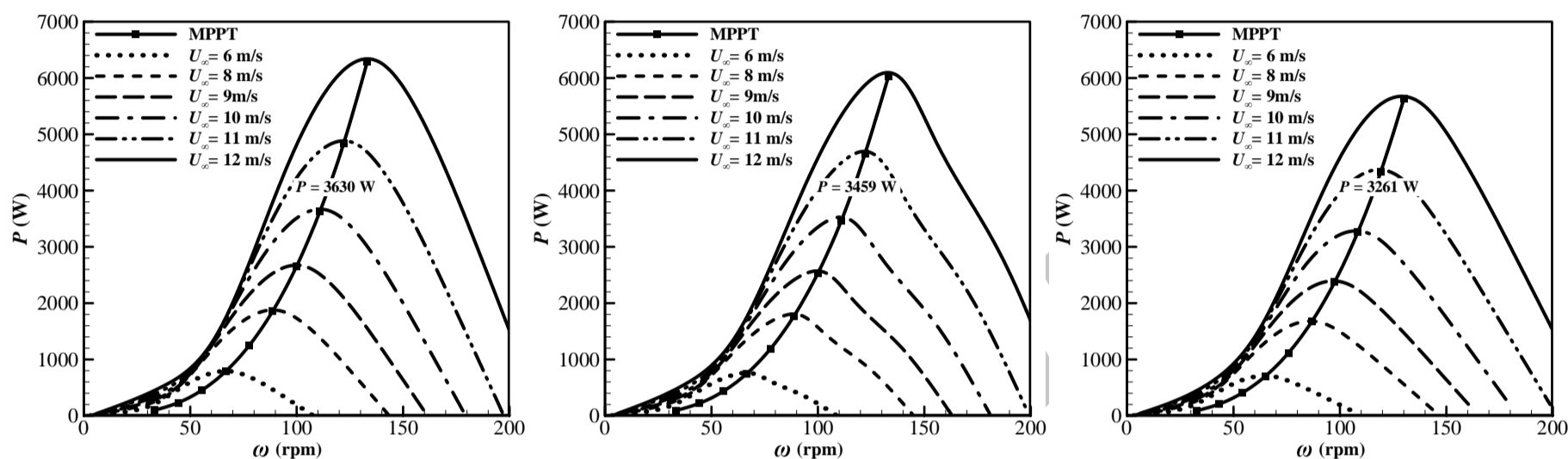
شکل 16 منحنی توان و MPPT برای پره با مقطع Du 13-J شکل 17 منحنی توان و MPPT برای پره با مقطع Du 23-J شکل 18 منحنی توان و MPPT برای پره با مقطع Du 33-J
