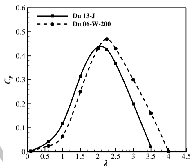
شکل 11 مقایسه منحنی عملکرد توربین با مقطع ل- Du 13-J و Du 06-W-200
