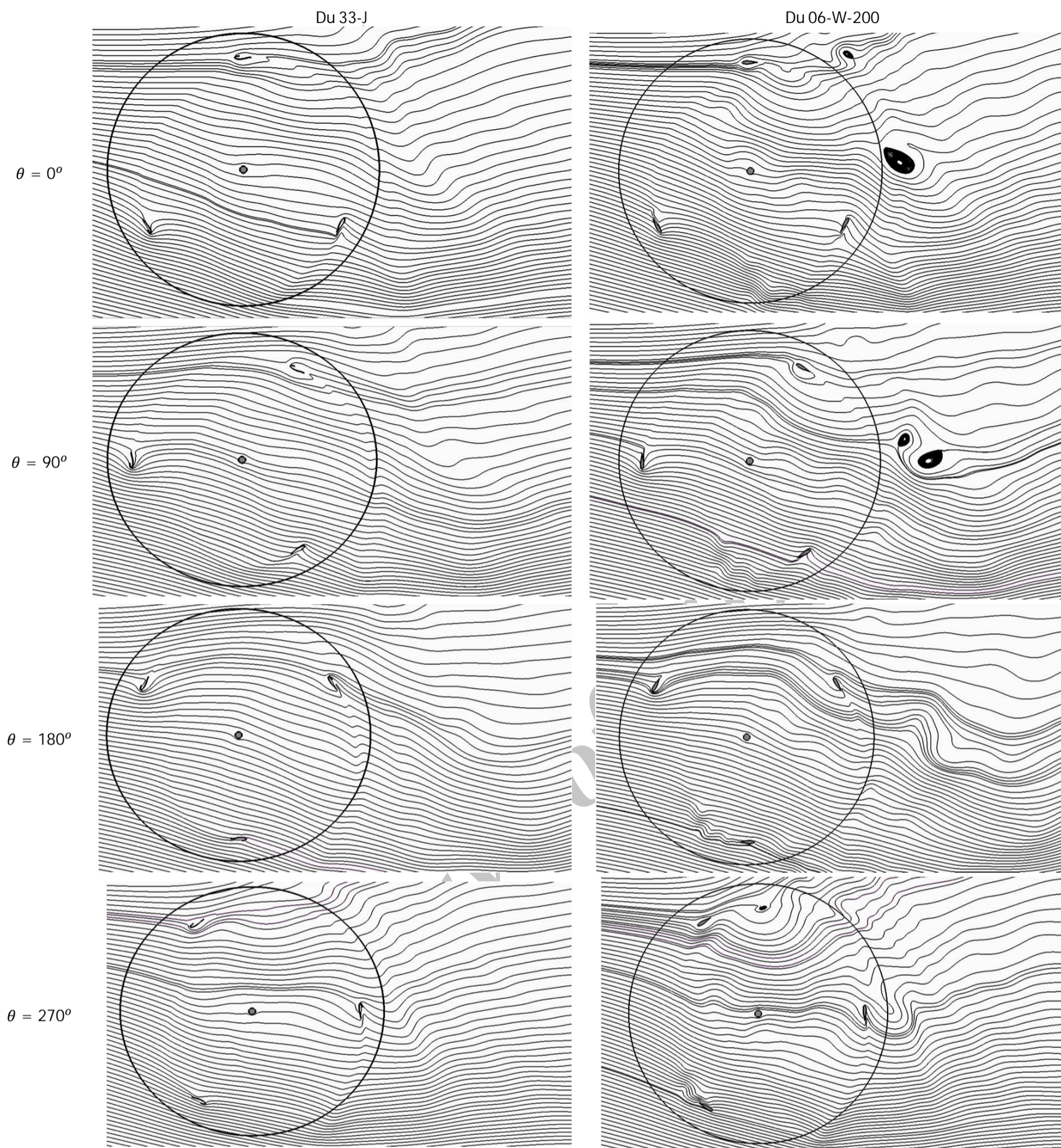
شکل 23 خطوط جریان حول روتور پس از رسیدن به حالت پایا در چهار زاویه چرخش از یک دوران کامل برای پره با ایرفویل Du 06-W-200 و Du 33-J در بهینه
