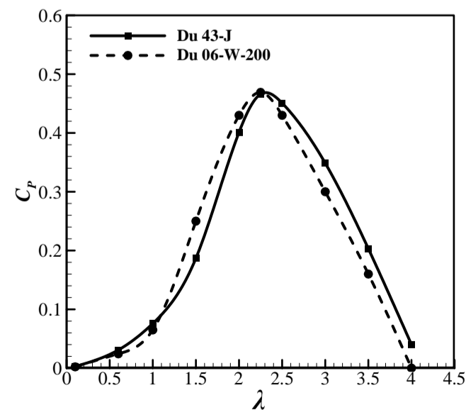
شکل 13 مقایسه منحنی عملکرد توربین با مقطع ل- Du 43-J و Du 06-W-200
