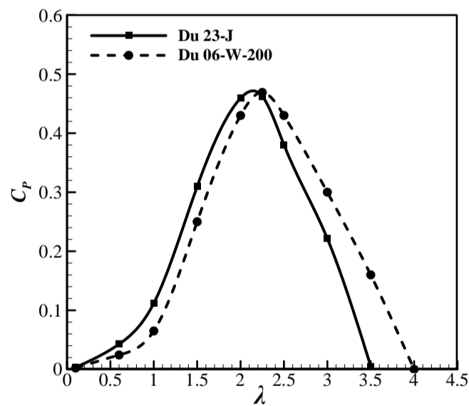
شکل 12 مقایسه منحنی عملکرد توربین با مقطع ل- Du 23-J و Du 06-W-200
