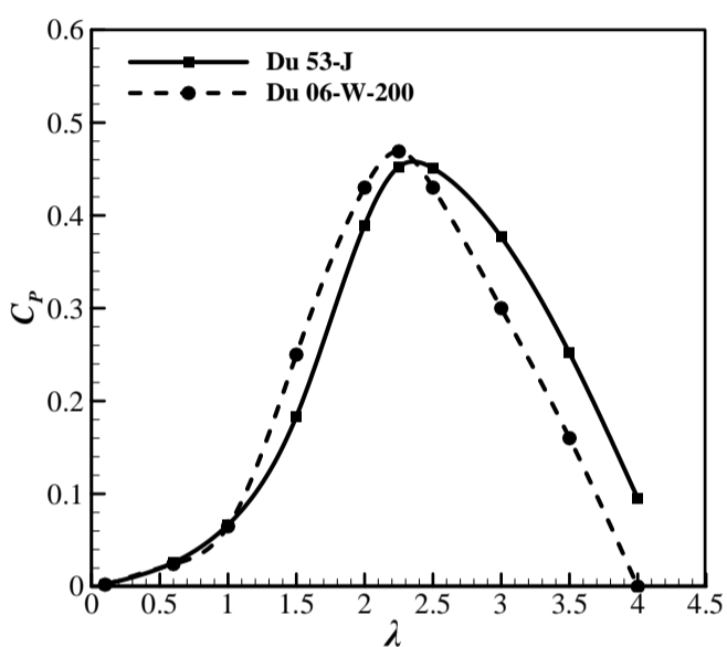
شکل 14 مقایسه منحنی عملکرد توربین با مقطع ل- Du 53-J و Du 06-W-200
