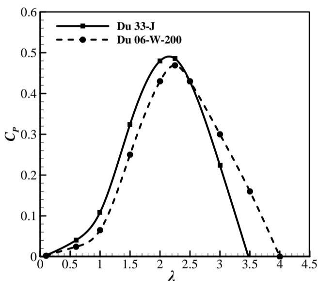
شکل 15 مقایسه منحنی عملکرد توربین با مقطع ل- Du 33-J و Du 06-W-200
