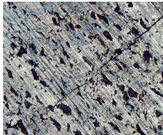
شکل 7 نمونه‌ای از سطح بزرگنمایی شده یک ترک واقعی در تیر که در آزمایشگاه مقاومت مصالح دانشگاه تبریز ایجاد شده است و با میکروسکوپ اولیمپوس \times 61 از آن تصویربرداری شده است.
