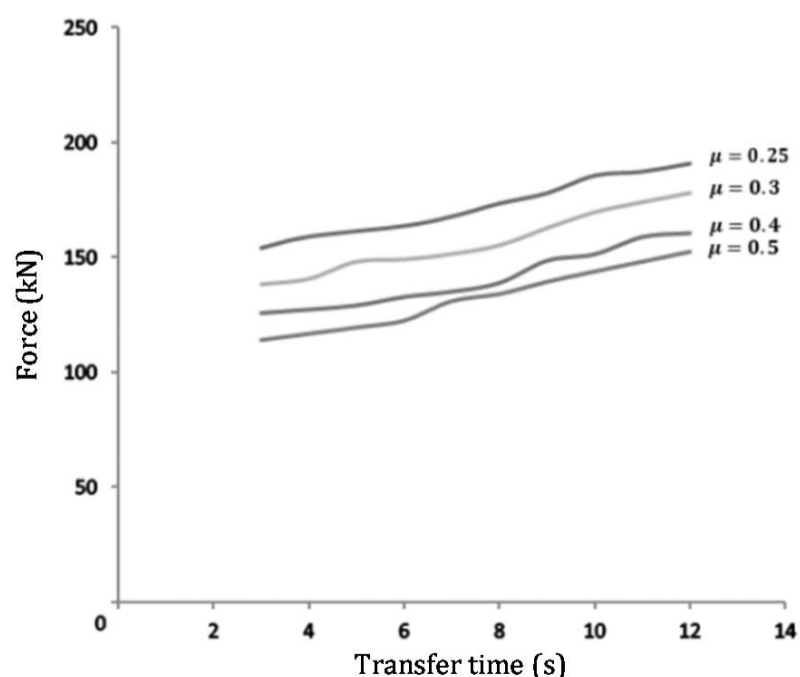
شکل 11 تاثیر اصطکاک در نیروی فرآیند اکستروژن پیش‌فرم پره در آزمایش‌های شبیه‌سازی شده
