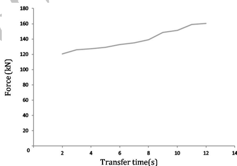
شکل 10 تغییرات نیروی فرآیند با افزایش زمان انتقال در طی آزمایش‌های شبیه‌سازی شده اکستروژن پیش‌فرم پره
