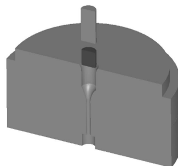
شکل 3 مدل شبیه‌سازی قالب، سنبه و بیلت
