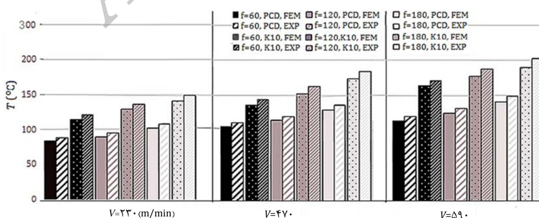
شکل ۷ توزیع درجه حرارت با تغییر سرعت برش و پیش‌روی برای PCD و K10 در نتایج عملی و شبیه‌سازی المان محدود
