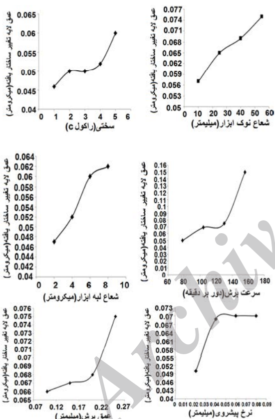
شکل ۱۱ نمودار اثر تغییر سختی قطعه کار (مدل ماده)، نرخ پیشروی ابزار، تغییر شعاع لبه ابزار و شعاع نوک ابزار و سرعت برش در تغییرات عمق لایه تغییر شکل یافته در شبیه‌سازی فرآیند ماشین کاری
